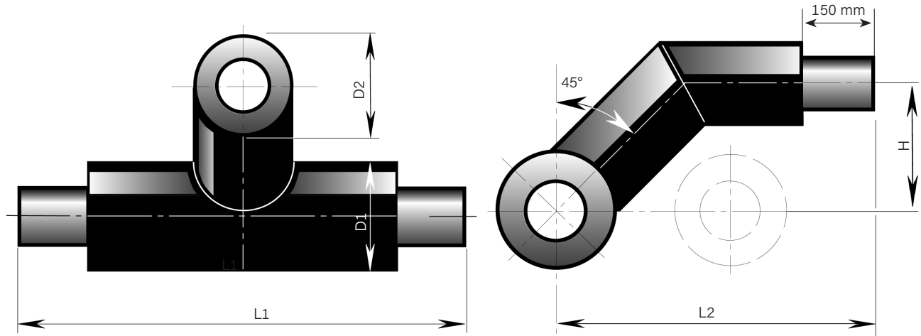
Dimensioni Ø 125 - 315 mm / SDR 11/ SDR 17
