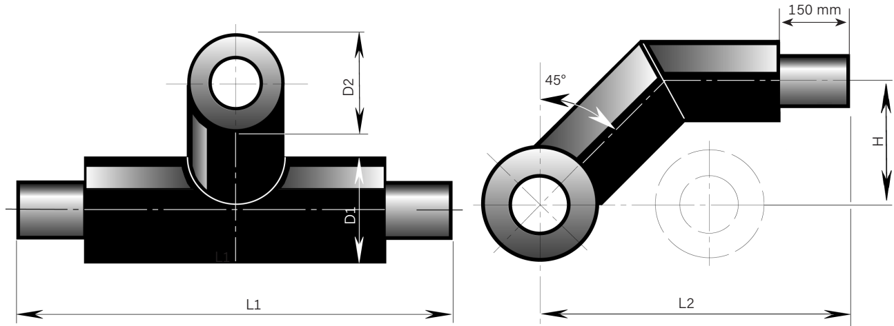
Dimensions Ø 125 - 315 mm / SDR 11/ SDR 17
